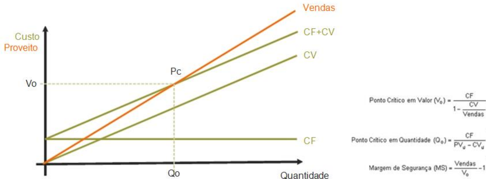
Figura 2: Dinâmica Custos
